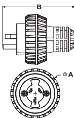
Phích Cắm Plug IP66 P-315
